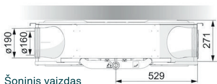
Šoninis vaizdas
