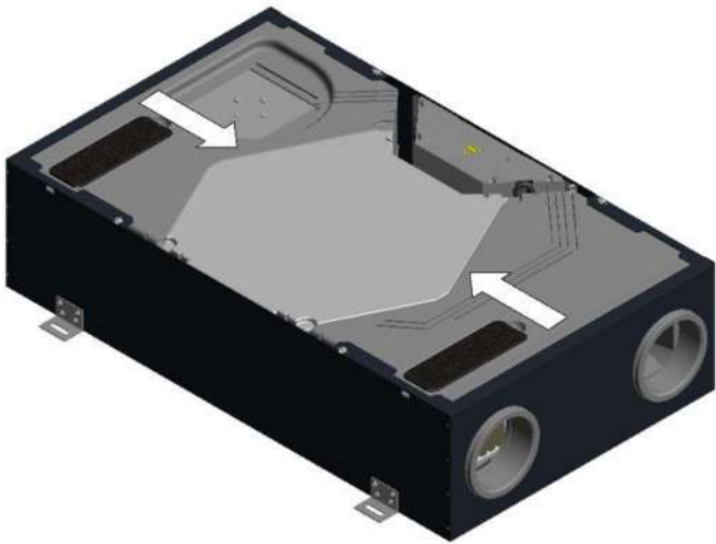
43 pav.: Ventilatorių dėžių pastūmimo kryptis užfiksavimui su šilumokaičio dėže
