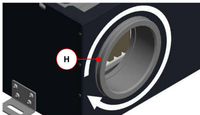
39 pav.: EPP jungės sutrumpinimas ties numatytąją atskyrimo vietą per juosiantį griovelį
