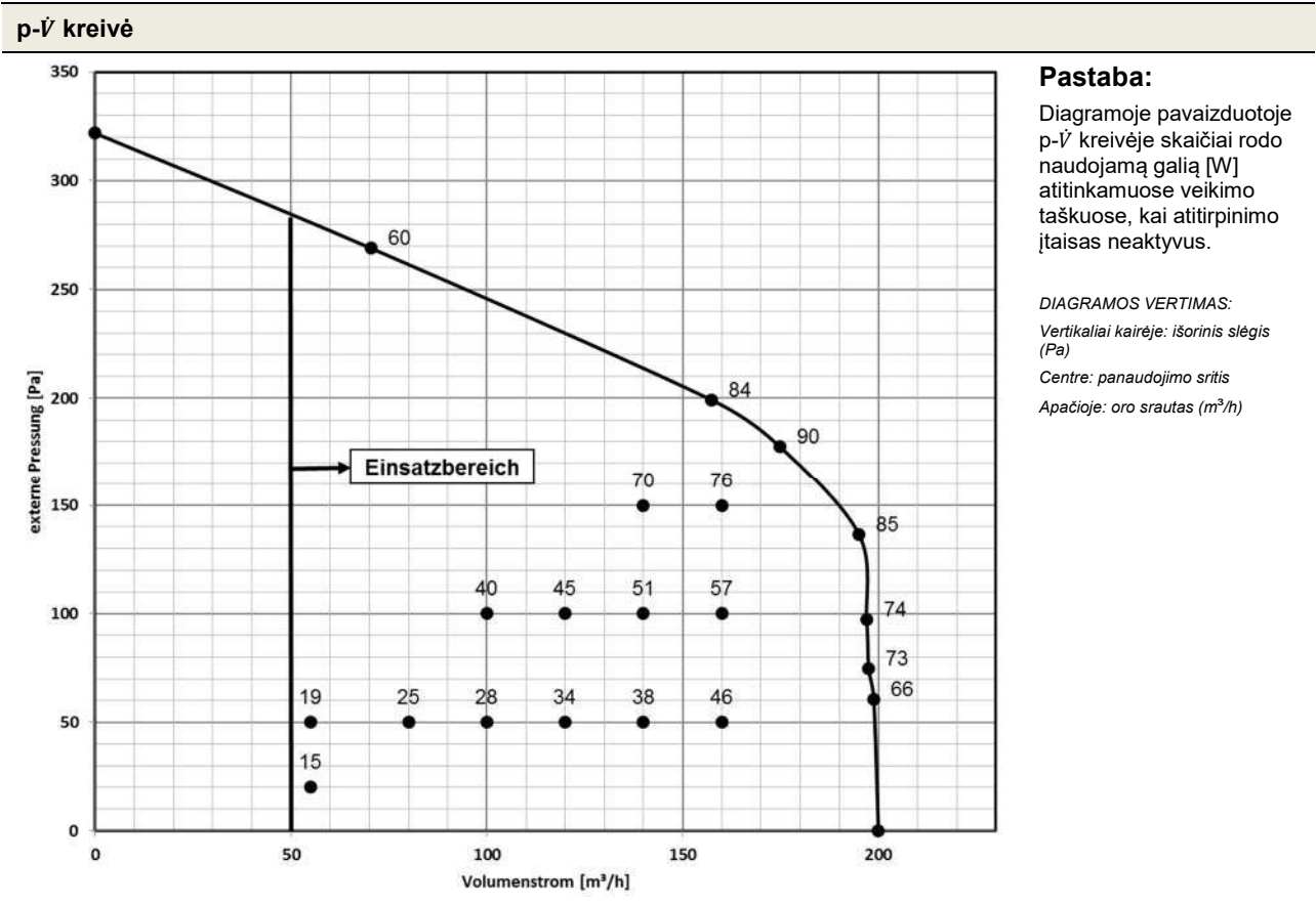
13 lent.: 3-a diagrama: „CLIMOS“ p-Ṽ kreivė
